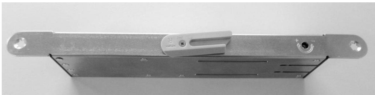
Pollmeier Drehmoment, Hebelarm in „Transportstellung“ (bzw. Geschlossen-Stellung)
