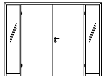
normalhoch mit Seitenteil, rechts und links als 1 bis 16 lieferbar
