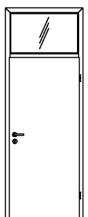
geschosshoch mit Oberlicht und Kämpfer
