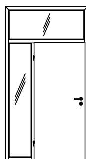
geschosshoch mit Oberlicht und Seitenteil, Tür am Pfosten angeschlagen
