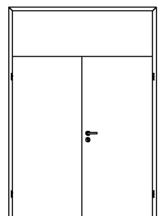
geschosshoch mit Blende als 1 bis 16 lieferbar
