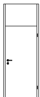
geschosshoch mit Blende, ohne Querstück, als 1 bis 16 lieferbar
