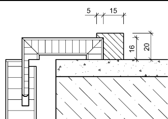
Wandanschlussleiste Typ P20
