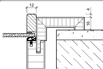
Glasleiste Typ O für gefälzte Zargen/Blendrahmen
