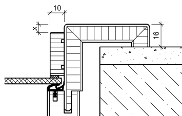
Glasleiste Typ S für stumpfe Zargen/Blendrahmen
