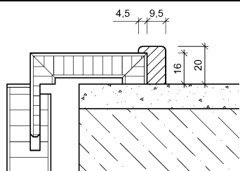
Wandanschlussleiste Typ L
