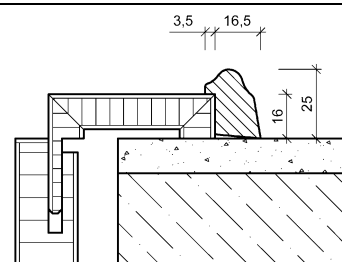
Wandanschlussleiste Typ B
