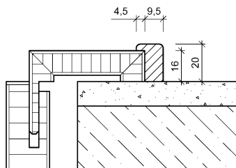
Wandanschlussleiste Typ L
