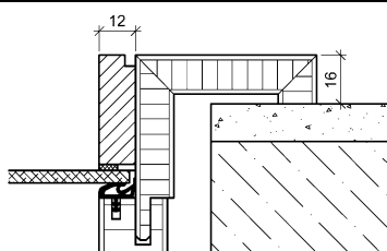
Glasleiste Typ Flächenbündig für stumpfe Zargen/Blendrahmen
