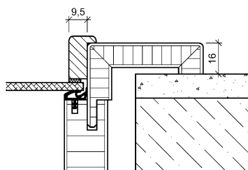
Glasleiste Typ L für gefälzte Zargen/Blendrahmen
