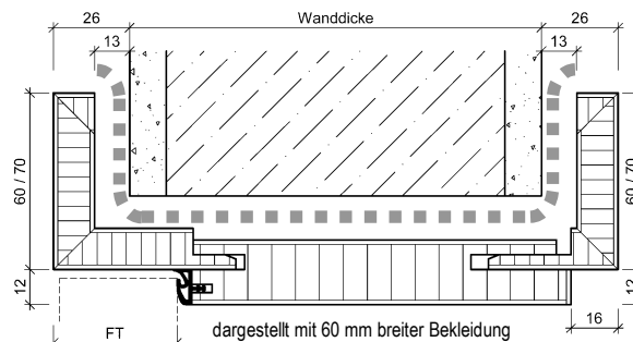
Renovierungs-Basis-Zarge B60 / B70 mit zusätzlicher Lüftungsfräsung im Bereich des Querstücks als Zu- oder Abluftöffnung, entstehender Lüftungsquerschnitt türbreitenabhängig: Türbreite 735 = ca. 78 cm 2 Türbreite 860 = ca. 91 cm 2 Türbreite 985 = ca. 104 cm 2
