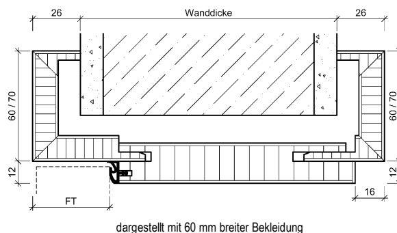
Renovierungs-Basis-Zarge B60 / B70 mit zusätzlicher Hobelnase, Bekleidung 26 mm auftragend, Oberflächen wie umseitig beschrieben
