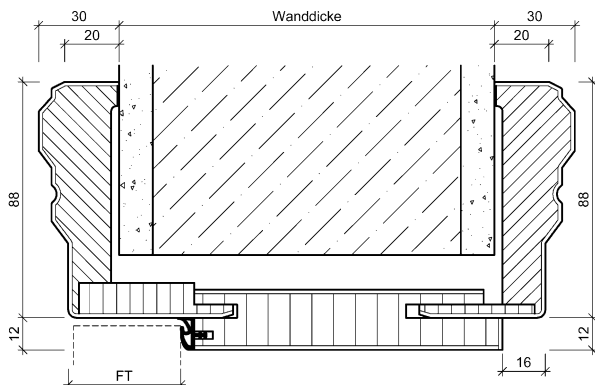
Basis-Zarge Ausführung „Klassik Line“ B88 Bekleidungsbreite 88 mm, ausschließlich farbig lackiert lieferbar
