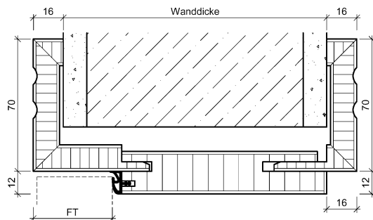
Basis-Zarge Ausführung „2 Rillen“ B70 Bekleidungsbreite 70 mm, ausschließlich farbig lackiert lieferbar
