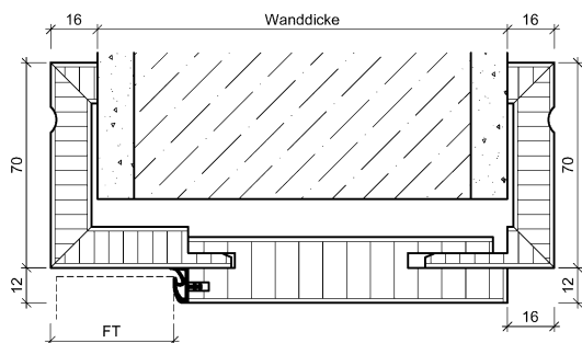
Basis-Zarge Ausführung „1 Rille“ B70 Bekleidungsbreite 70 mm, ausschließlich farbig lackiert lieferbar
