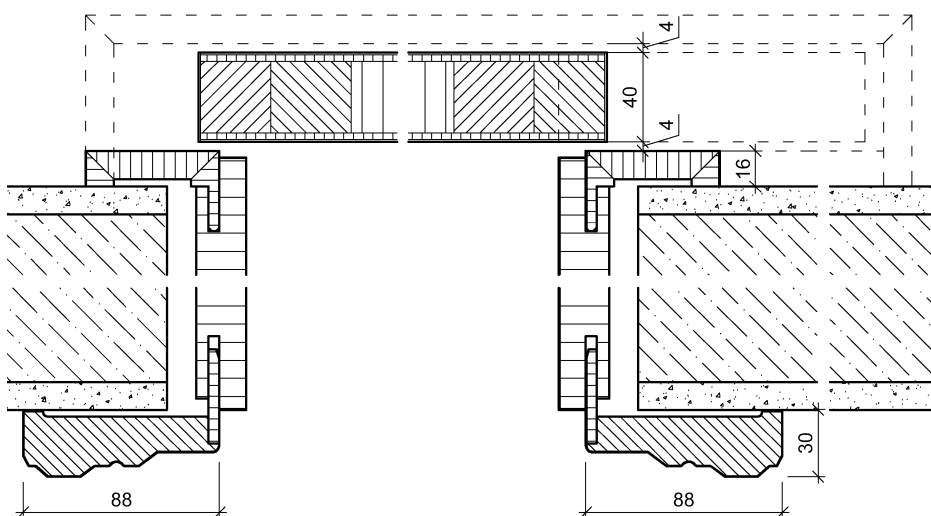
Basis-Schiebetürzarge vor der Wand laufend, Ausführung „Klassik Line“ B88 (nur bei farbig lackierten Oberflächen möglich)
