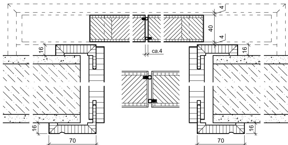
Basis-Schiebetürzarge vor der Wand laufend, Ausführung „1 Rille“ B70 (nur bei farbig lackierten Oberflächen möglich)
