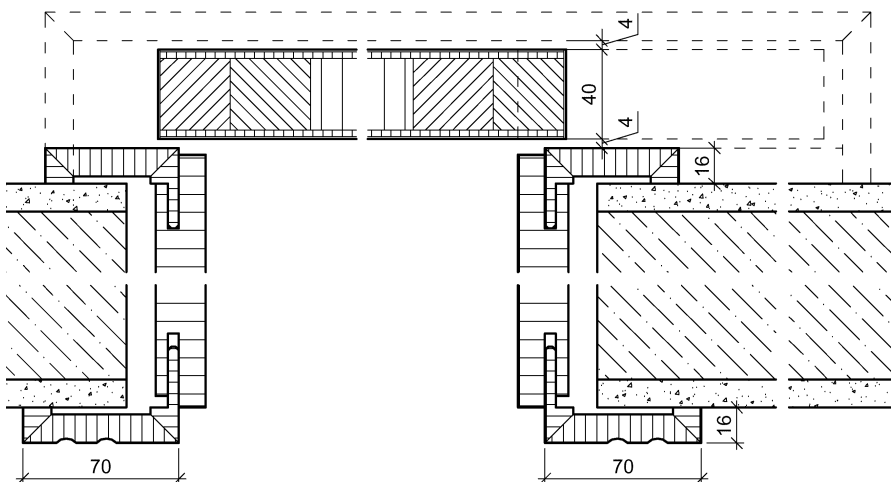
Basis-Schiebetürzarge vor der Wand laufend, Ausführung „2 Rillen“ B70 (nur bei farbig lackierten Oberflächen möglich)
