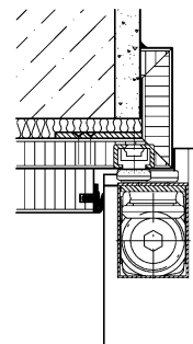
verdeckt liegender Türschließer
