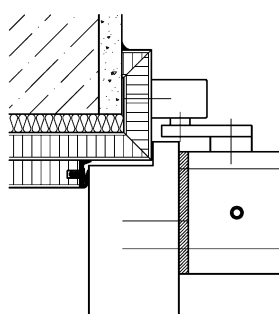
Gleitschienen-Türschließer in Normalmontage
