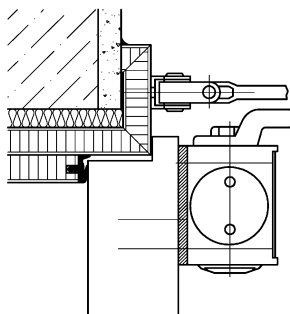
Scherenarmtürschließer in Normalmontage (Standard)
