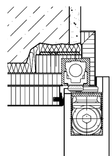
verdeckt liegender Türschließer mit elektrome- chanischer Feststellung
