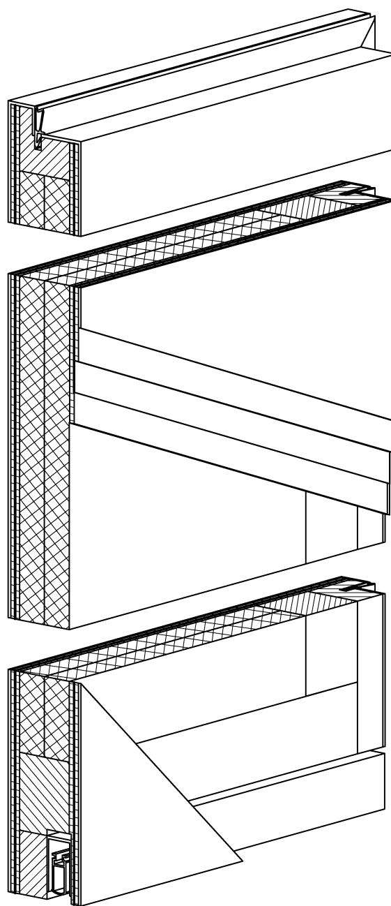
Schallschutztür 45 WE-SK3, gefälzt, (dargestellt mit Aluminium Verbundabsperung für Klimaklasse III)
