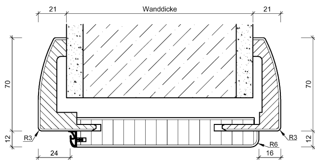
Rund-Zarge „Softline“ B70 ausschließlich farbig lackiert lieferbar und in CPL Weißlack ähnl. 9010
