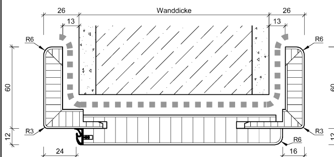
Rund-Renovierungszarge B60 mit zusätzlicher Lüftungsfräsung im Bereich des Querstücks als Zu- oder Abluftöffnung, entstehender Lüftungsquerschnitt türbreitenabhängig: Türbreite 735 = ca. 78 cm 2 Türbreite 860 = ca. 91 cm 2 Türbreite 985 = ca. 104 cm 2
