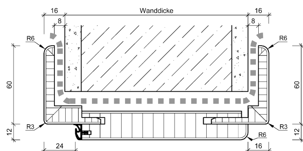
Rund-Zarge B60 mit zusätzlicher Lüftungsfräsung im Bereich des Querstücks als Zu- oder Abluftöffnung, entstehender Lüftungsquerschnitt türbreitenabhängig: Türbreite 735 = ca. 48 cm 2 Türbreite 860 = ca. 56 cm 2 Türbreite 985 = ca. 64 cm 2
