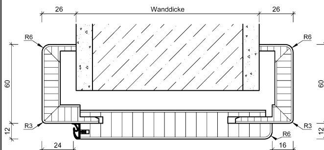
Rund-Renovierungszarge B60, ausschließlich farbig lackiert lieferbar und in CPL Weißlack ähnl. 9010
