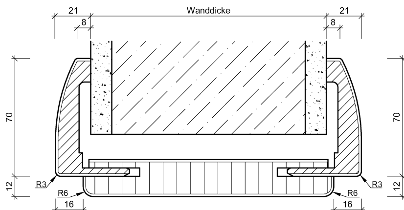
Rund-Durchgangszarge „Softline“ B70 ausschließlich farbig lackiert lieferbar und in CPL Weißlack ähnl. 9010
