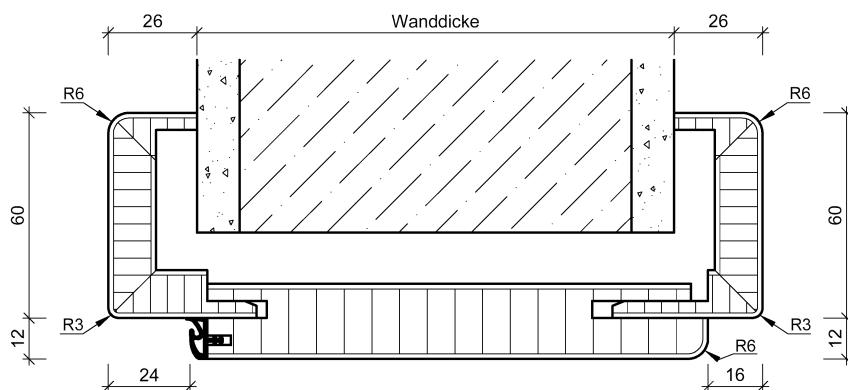
Rund-Renovierungszarge B60 mit zusätzlicher Hobelnase, Bekleidung 26 mm aufragend, ausschließlich farbig lackiert lieferbar und in CPL Weißlack ähnl. 9010
