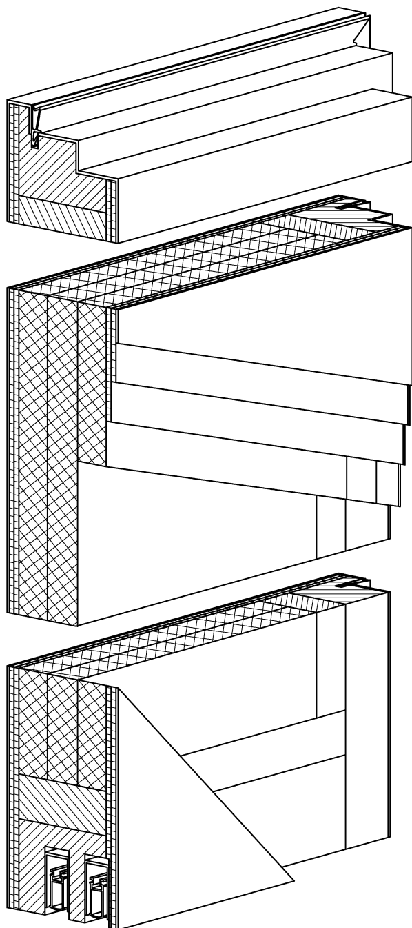
Schallschutztür 70 WE-SK4 mit Doppelfalz
