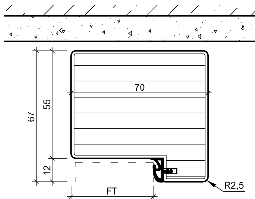
Bild 4 , montiert in der Wand
