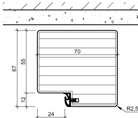
Bild 2, montiert in der Wand
