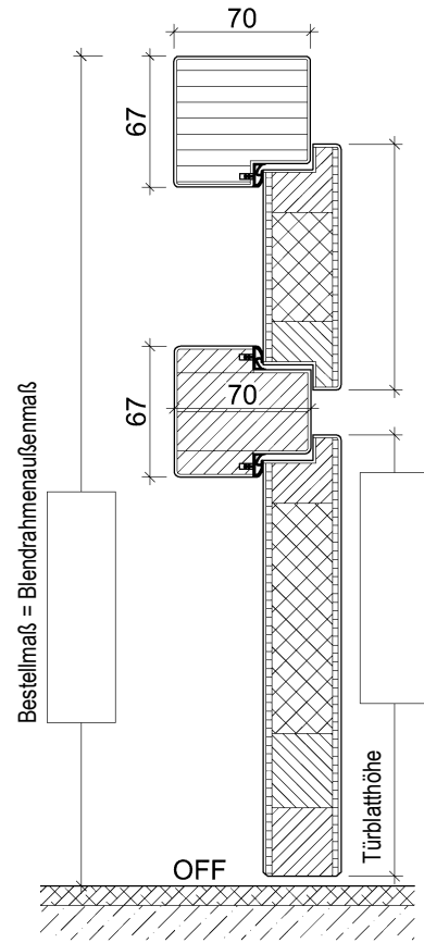
Bild 2 Oberblende mit Kämpfer
