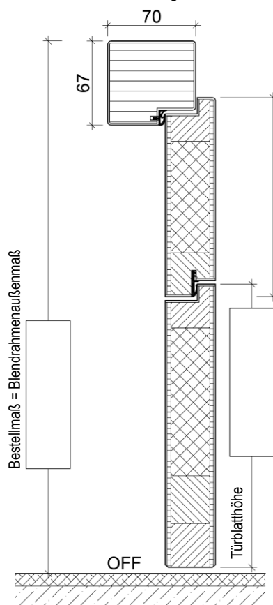
Bild 1 Oberblende mit Gegenfalz
