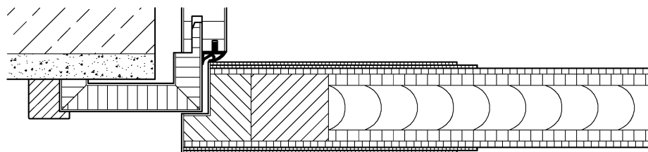
Wohnraumtür Classique Nouveau 1, Variante A mit geradem Aufschlag, mit Basis-Zarge B70, mit Wandanschlussleiste P20, gefälzt
