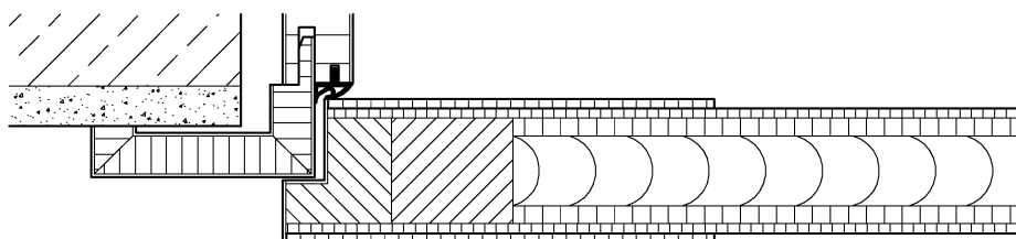
Wohnraumtür Classique Nouveau 1, mit geradem Aufschlag, mit Basis-Zarge B70, gefälzt
